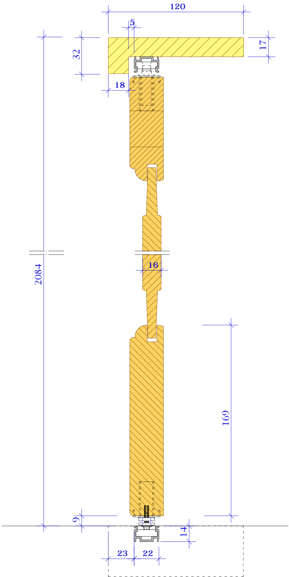
SECTION 1:2 Atle
